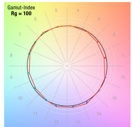
FARBTONVERSCHIEBUNG – TM-30
