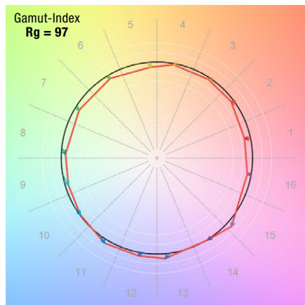
FARBTONVERSCHIEBUNG – TM-30
