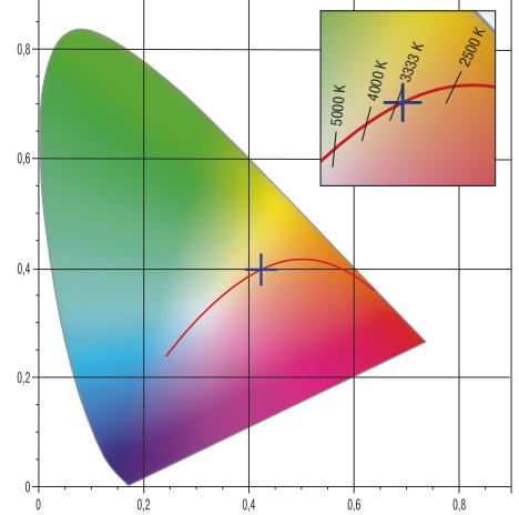
FARBWIEDERGABE – TM-30
